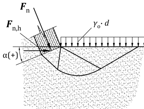
a) positiver Sohlneigungswinkel
