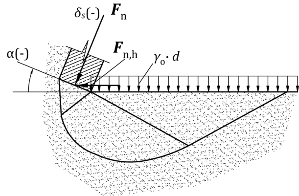
b) negativer Sohlneigungswinkel
