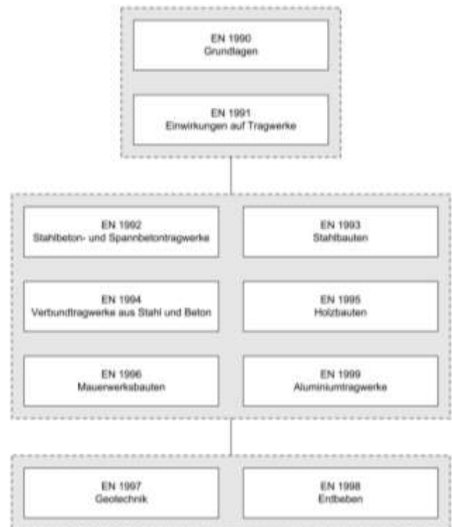
Bild 4: Struktur der Eurocodes
